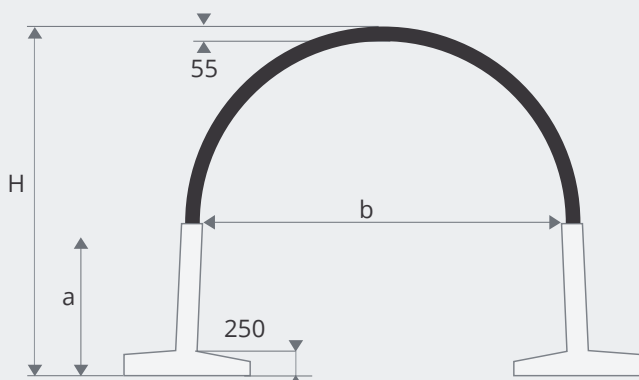
Kuva 1: Rakennemitat
